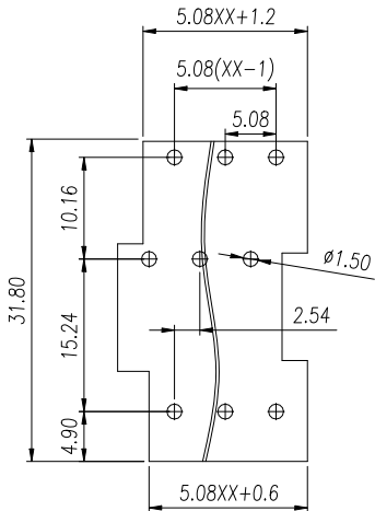
P.C.B. LAYOUT
